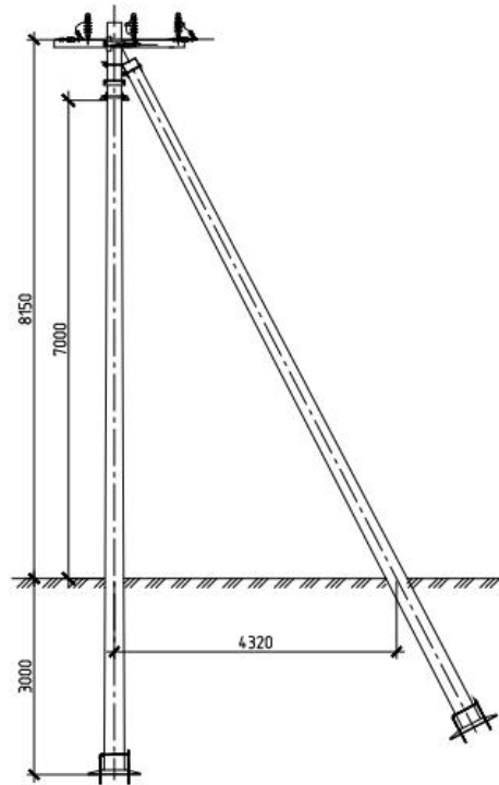
Угловая анкерная опора ОУА10-11
