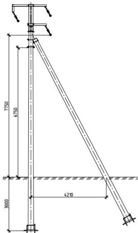
Угловая промежуточная опора ОУП10-11п
