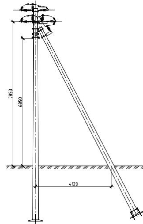
Угловая ответительная анкерная опора ОУОА10-11
