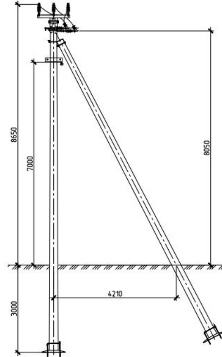
Ответительная анкерная опора ООА10-11
