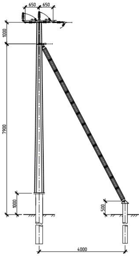
Анкерно-угловая свободностоящая опора АУ10Ф-2СР
