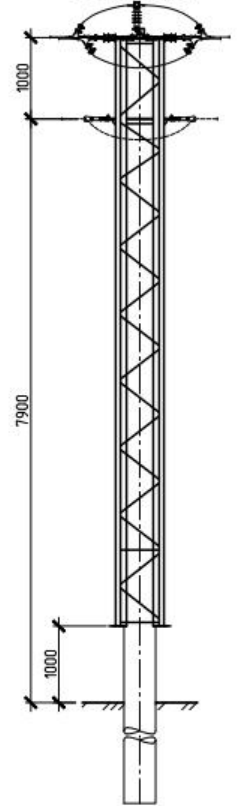
Анкерная свободностоящая опора АС10Ц-ЗСР
