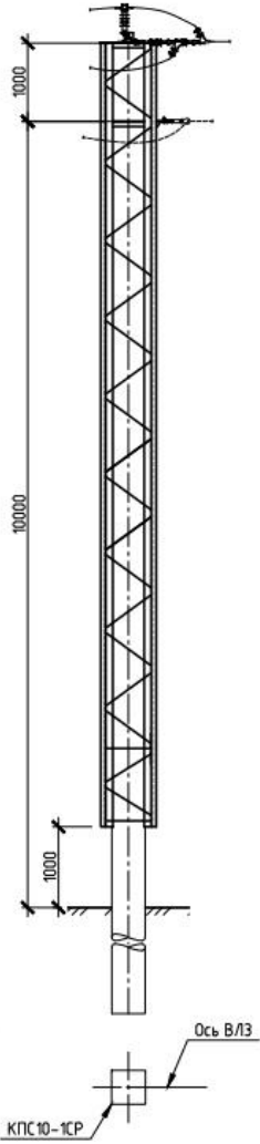
Концевая поышенная свободнотящая опора КПС10Ц-1СР
