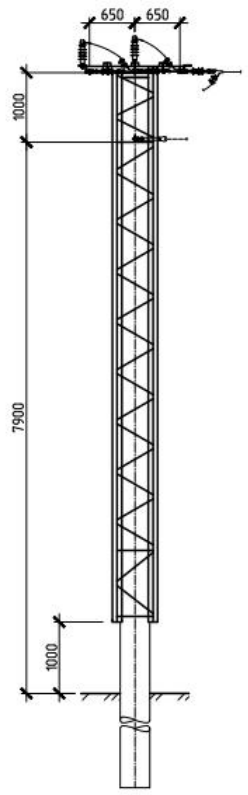
Анкерно-угловая свободностоящая опора АУС10Ц-2СР
