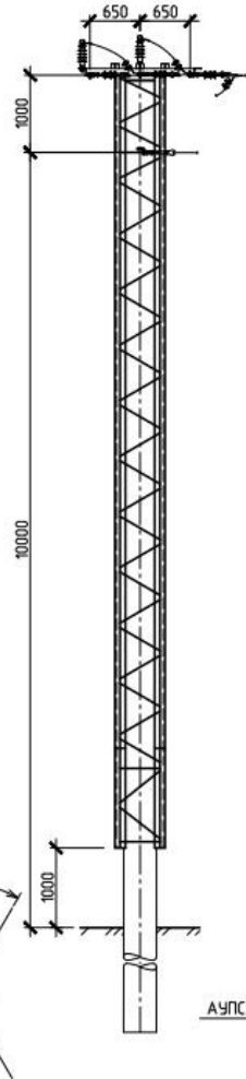
Анкерно-угловая поышенная свободнотящая опора АУПС10Ц-1СР
