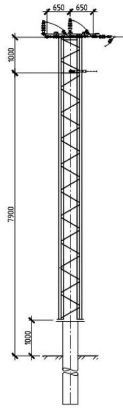
Анкерно-угловая свободностоящая опора АУС10Ф-2СР
