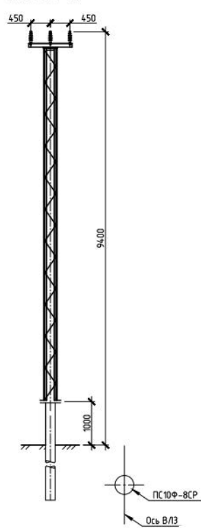
Промежуточная свободностоящая опора ПС 10Ф-8СР
