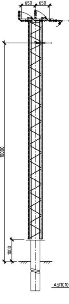
Анкерно-угловая поышенная свободнотящая опора АУПС10Ф-1СР
