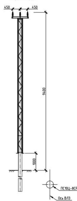
Промежуточная свободностоящая опора ПС 10Ц-8СР
