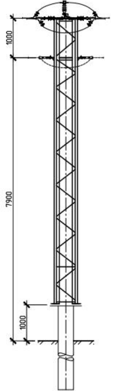
Анкерная свободностоящая опора АС10Ф-ЗСР
