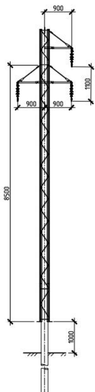
Промежуточная свободностоящая опора ПС 10Ц-10СР
