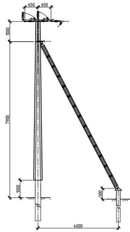
Анкерно-угловая свободностоящая опора АУ10Ц-2СР
