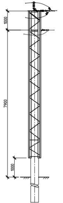
Концевая свободностоящая опора КС10Ц-ЗСР
