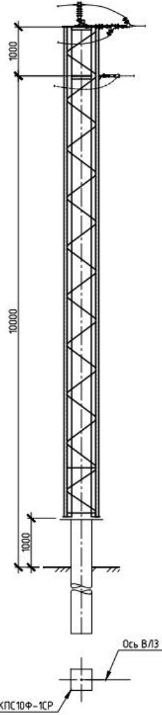
Концевая поышенная свободнотящая опора КПС10Ф-1СР
