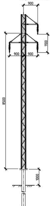
Промежуточная свободностоящая опора ПС 10Ф-10СР
