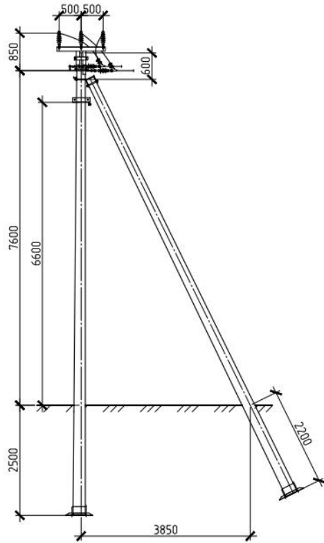
Ответвительная анкерная опора 00А10-10.5
